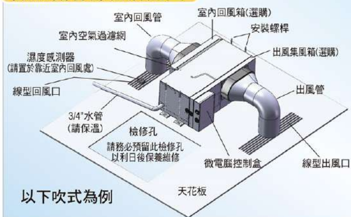
除濕機各部位解說圖
