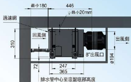
TSD-140N 安裝示意圖
